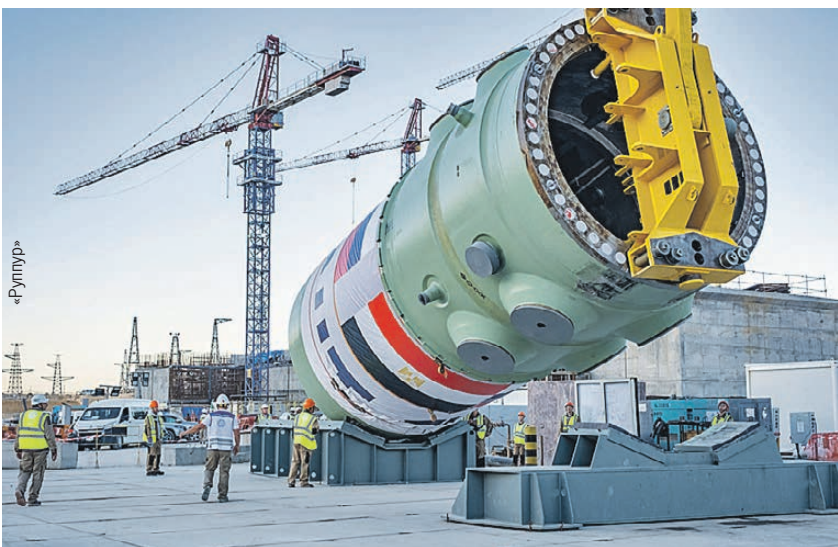
В Египте установили в проектное положение корпус реактора первого энергоблока АЭС «Эль-Дабаа».
